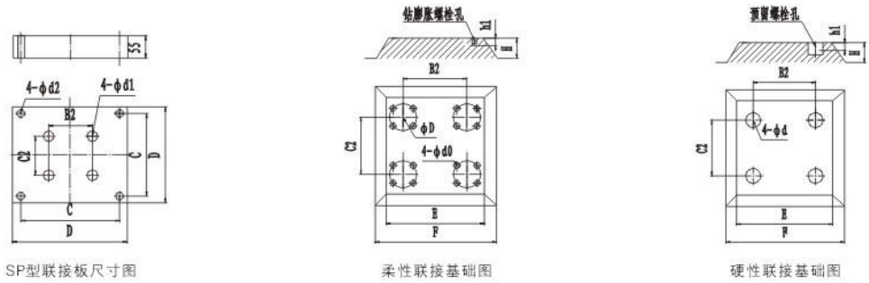
SP型联接板尺寸图
